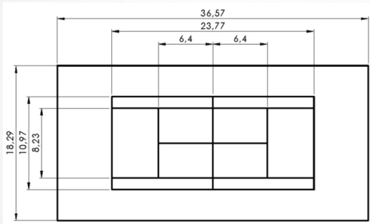
Dimensões oficiais de uma quadra de Tênis
